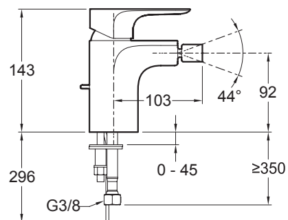
E72279-** E72350-**
