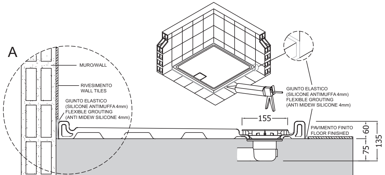
INSTALLAZIONE SOPRA AL PAVIMENTO (IN APPOGGIO) SURFACE-MOUNTED INSTALLATION
