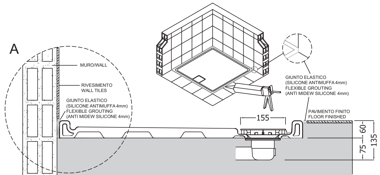
INSTALLAZIONE FILO PAVIMENTO (INCASSO) FLUSH WITH FLOOR INSTALLATION
