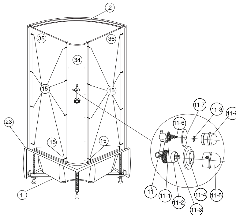
Схема установки центральной и задних панелей
